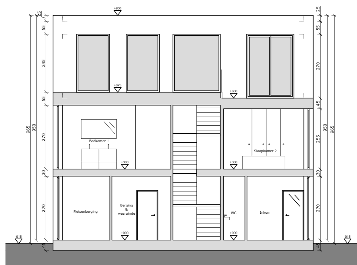
Doorsnede CC'
