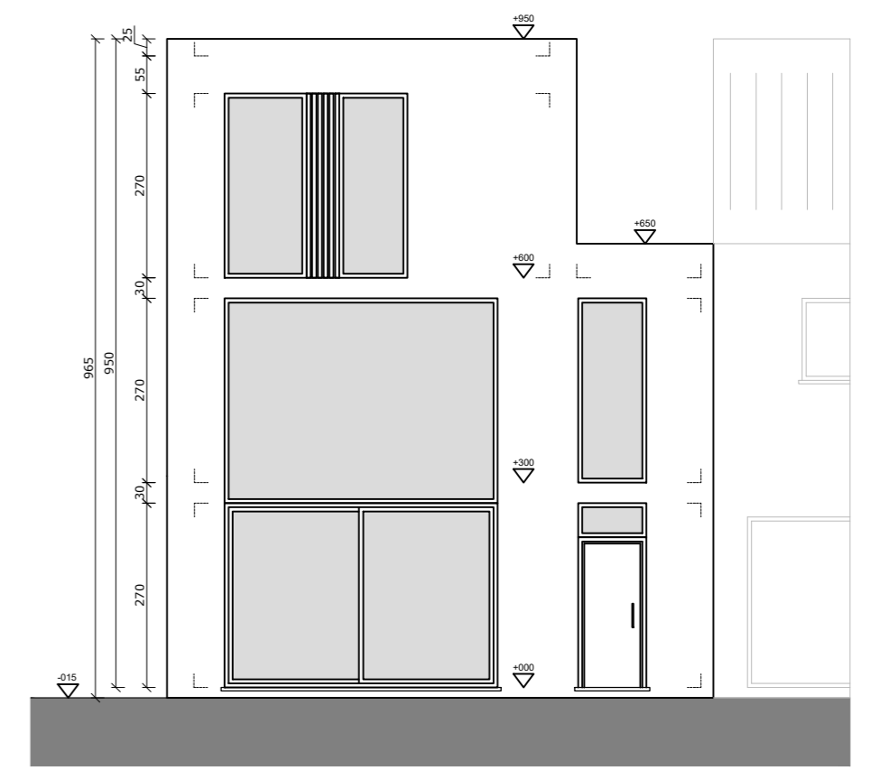
Achtergevel
