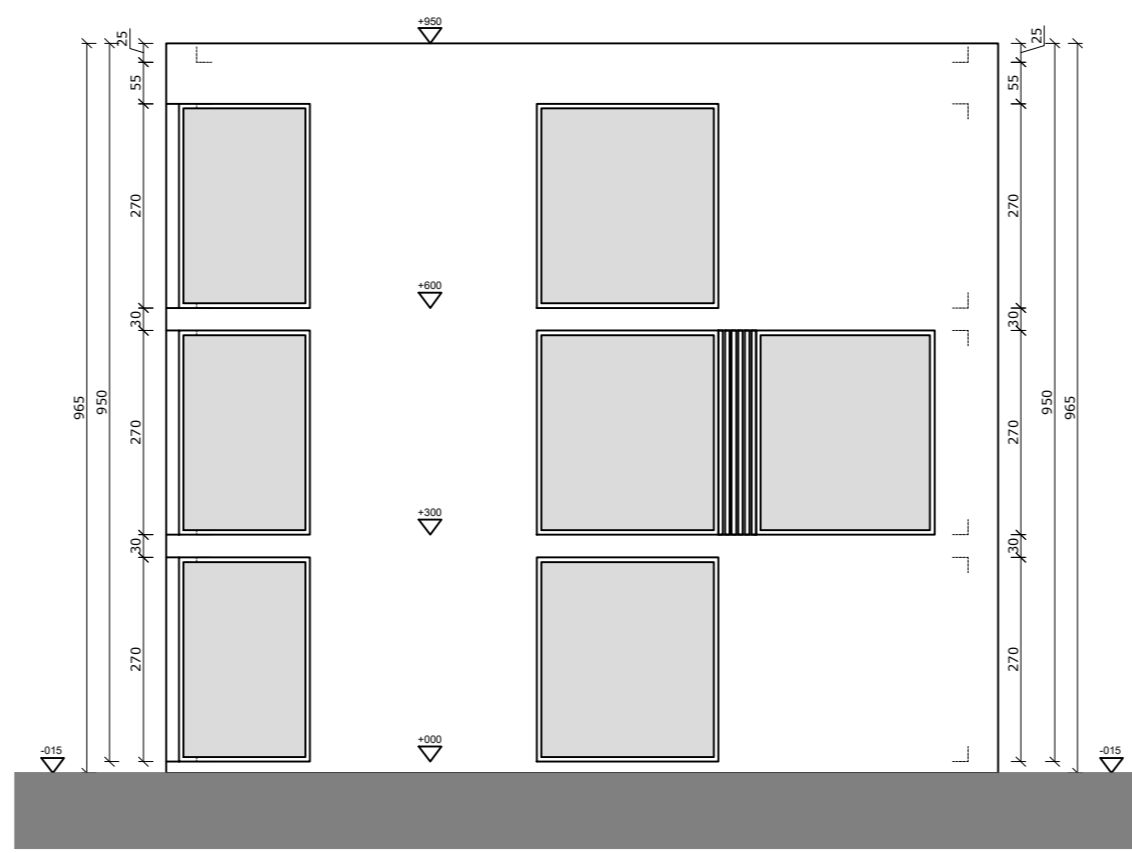
Rechterzijgevel
