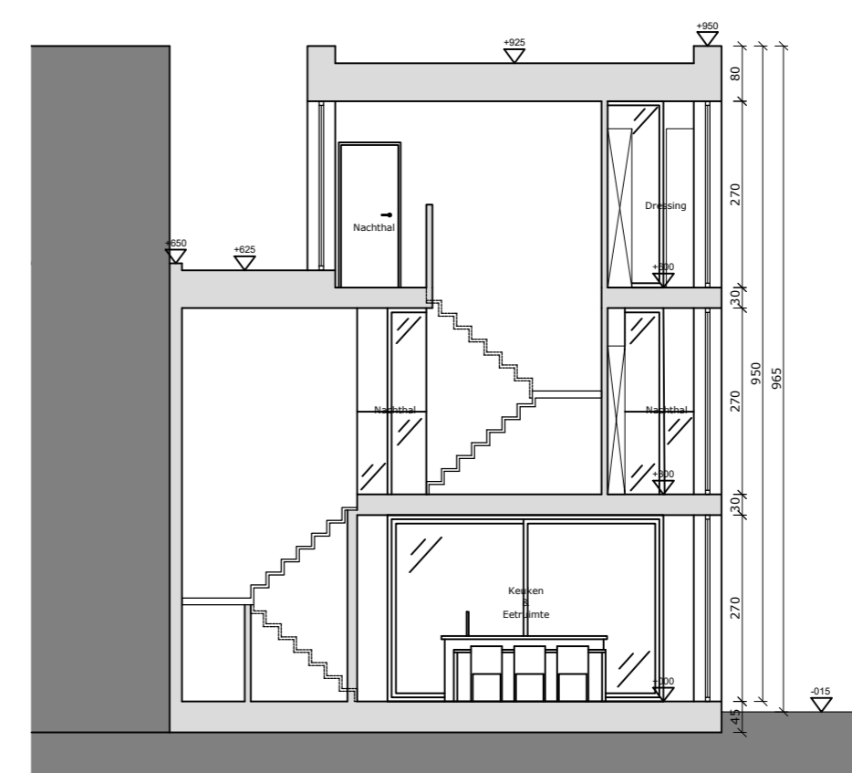
Doorsnede BB'
