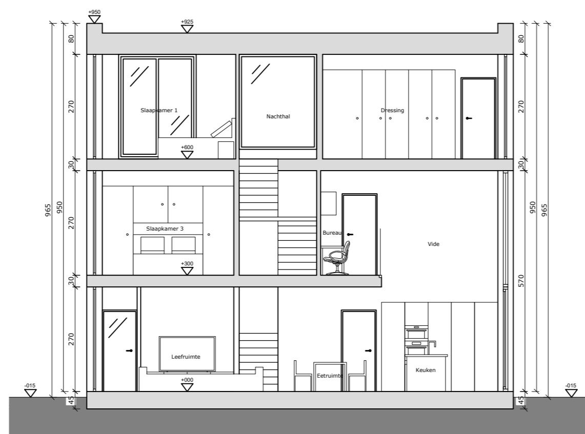
Doorsnede AA'
