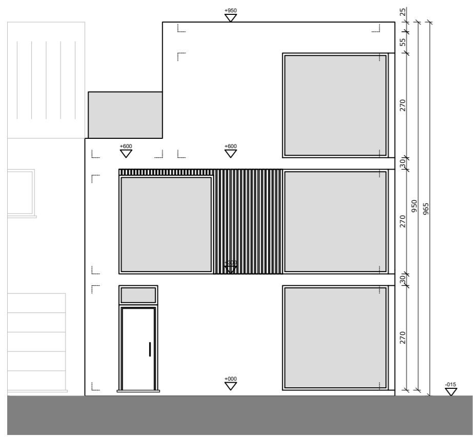
Voorgevel
